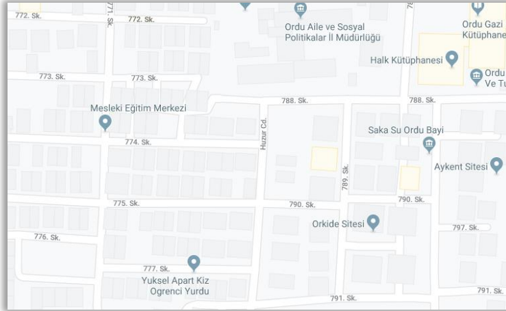
Şekil 2.Ordu ili, Altınordu ilçesi Akyazı mahallesine ait sokak haritası (Anonim 2)
